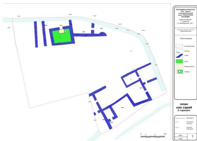
2-сызба – Хан Ордасы екінші құрылыс қабатының жобасы
